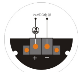
2线制接线图
